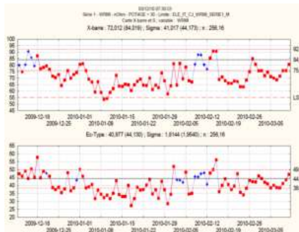
rysunek: Karta \bar{x} -średnie i s opisującą proces związany z elektrolizą aluminium
